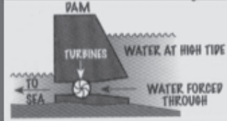
టైడల్ విద్యుత్తు
