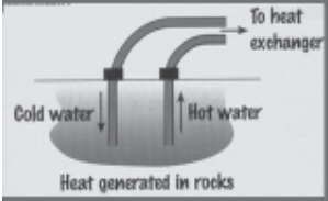
జియోథర్మల్ విద్యుత్తు
